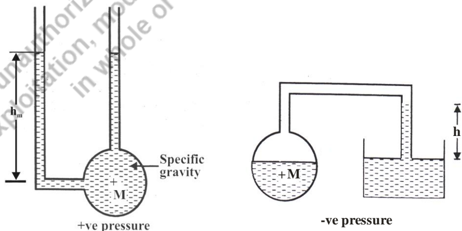
Fig. 2.7 Piezometer
